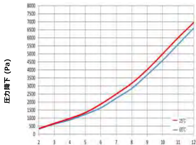
冷却水流量 (L/min.) 図 2: 圧力降下と冷却水流量
