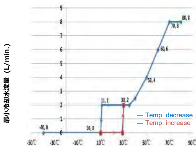
冷却水温度 図 1: 最小冷却水流量と冷却水温度
