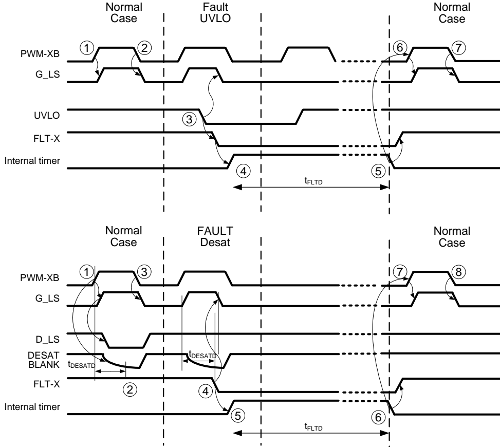
図24：タイミング図 CMT-PLA3SA12450A ローサイドゲートドライバの動作
